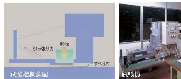
INAXの滑り試験 (東工大式すべり試験機)
